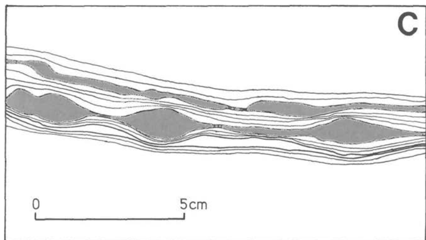
◄▲ Abb. 6. Boudinage-Gefüge im Massenkalk als Ergebnis einer ausgeprägten Dehnung in Richtung des tektonischen Transportes (a). – Steinbruch in der Glinne (1). A: Kompetente feinschichtige Dolomit-Boudins getrennt durch calcitische Zwickelfüllung (punktiert) und umhüllt von stärker duktilem, tektonisch laminierten Massenkalk. B: Rotierter feinschichtiger Dolomit-Boudin. Streckungshöfe mit Calcit (punktiert) gefüllt. C: Pinch-and-swell structure in dolomitischen Lagen. Die beginnende Trennung kompetenter Lagen stellt die Vorstufe der Boudinierung dar.
