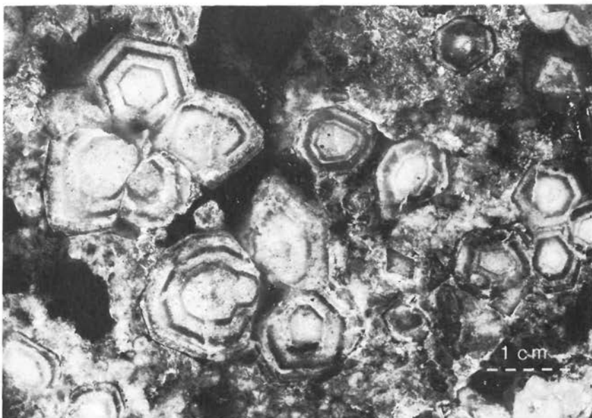
Abb. 3. Dichte Kristallpackung Suttruper Quarze (Zonarbau) in sekundär verkieseltem Gangmaterial (mit Pseudomorphosen nach Dolomit); vgl. H. BEHR et al. (1979). Sammlung Wiemeyer.
