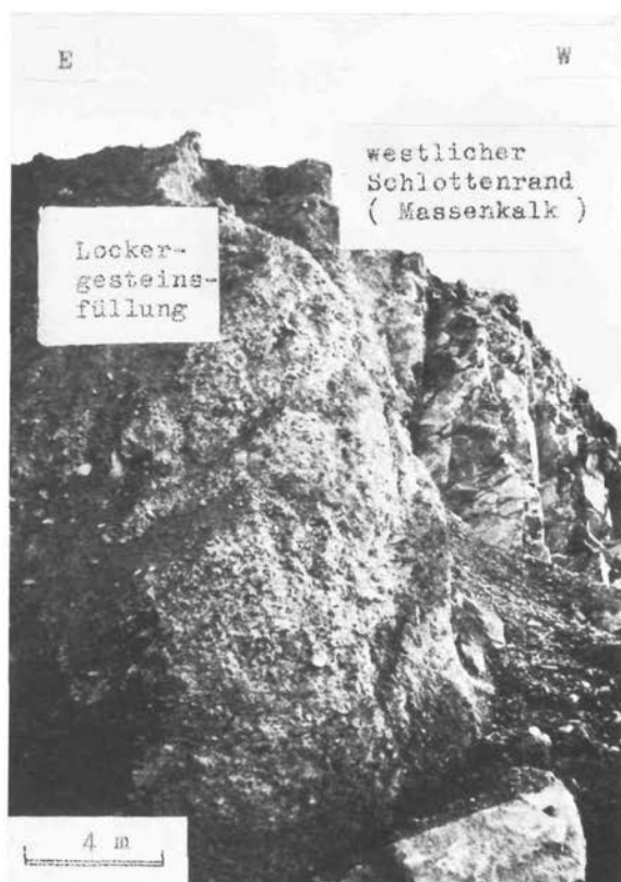
Abb. 2. Massenkalk-Steinbruch Brühne/Hillenberg, Südostwand (R 55 730, H 00 090). Übersicht über die aus unterschiedlich großen Komponenten zusammengesetzte Lockergesteinsfüllung der Karstschlote. Nach Westen Übergang in den aus Massenkalk bestehenden Schlottenrand.
