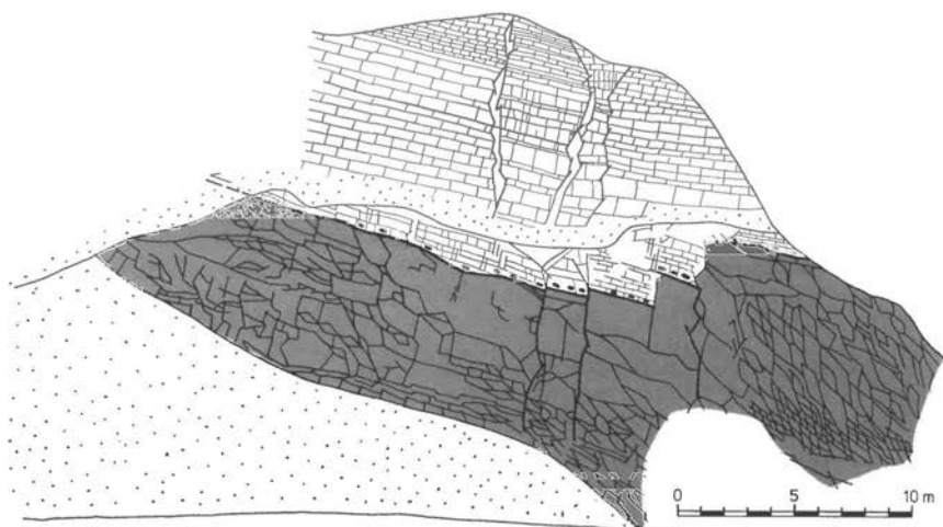
Abb. 8. Kulmkieselschiefer und höchste Abschnitte der Liegenden Alaunschiefer (mit Phosphoritknollen) überfahren an flacher Überschiebungsbahn die phacoidisierte Folge der Flinschiefer und Flinskalke der Adorf-Stufe. – Steinbruch am Kalvarienberg (10).
