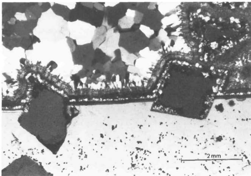
Abb. 4. Randzone eines Quarzgroßkristalls mit eingewachsenen Dolomithkristallen, die sekundär dedolomitiert wurden und jetzt als Negative vorliegen. Kleine Hämatitrosen innerhalb des Quarzkristalls (schwarze Pünktchen). Jüngerer Chalzedon umwächst den Quarzkristall und Dolomit. Darüber Quarzabscheidungen in Kornmosaiken (links oben); Radlinghausen.
