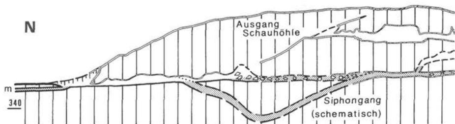
Abb. 14. Längsprofil (teilweise etwas schematisch) durch das Bilstein-Höhle-System (nach Vermessungen von F. HEINE (1931) und einem Entwurf von J. DOLLE/Warstein, ergänzt und umgezeichnet).
