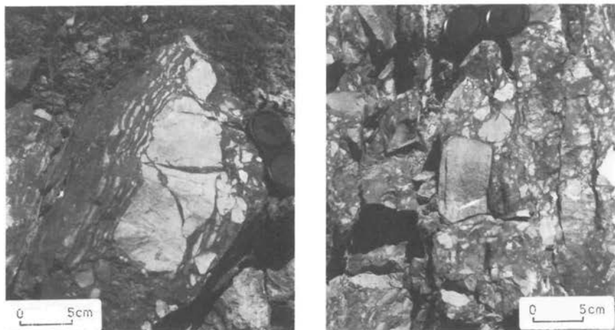
Abb. 3. Schlagwasser-Brekzie. Polymikte Brekzie aus Cephalopoden- und Flinzkalken in einer unterkarbonischen tonig-mergeligen Matrix. – Straßenanschnitt S Kallenhardt (7).
