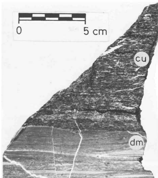
Abb. 4. Spaltenfüllung aus unterkarbonischem Crinoiden-Kalk (Erdbacher Kalk, cu) im Massenkalk (dm). Spaltenfüllung und Massenkalk sind intensiv tektonisch ausgelängt bzw. miteinander verschleift. – Steinbruch in der Güns (1).
