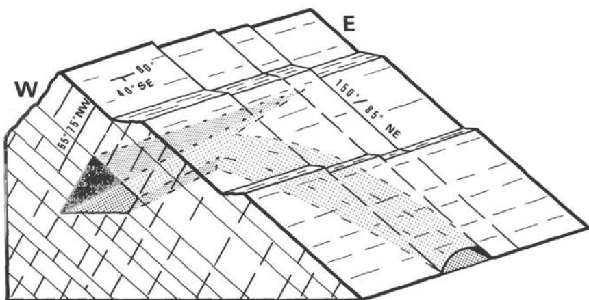
Abb. 22. Hohlraumbildung und Tektonik, Strukturschema des Hohlen Steins.
