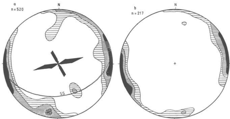
Abb. 12. Sammel-Polpunktdiagramme aus Massenkalk-Steinbrüchen Warsteins. a) Klüfte, unverkarstet; ss-Großkreis \Delta Maximum der Schichtflächenpole; Richtungsrose: Störungen. b) Karsthohlformen, vor allem Spalten.
