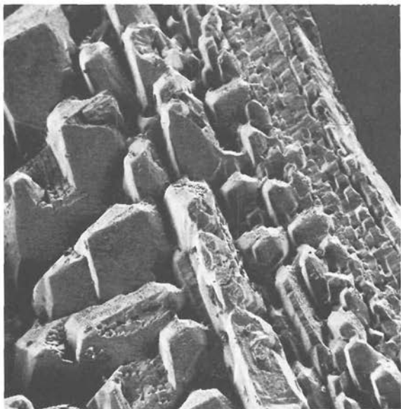
Abb. 7. Parallele Anlagerung von Rhomboederflächen (Ausschnitt aus Abb. 6). Bildbreite 0,52 mm. (REM-Aufnahme).
