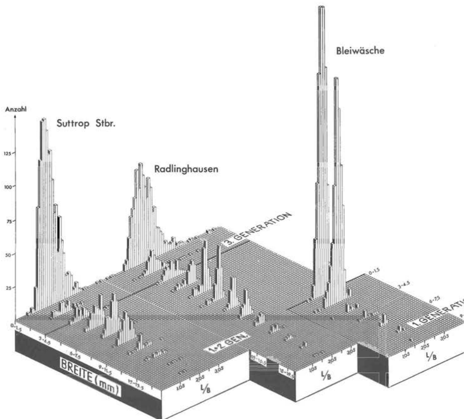
Abb. 7. Zusammenstellung der computerstellten dreidimensionalen Häufigkeitsverteilungen nach der Breiten-Klasseneinteilung. Nach oben ist die absolute Häufigkeit der Quarze in Abhängigkeit von der Breite und dem Quotienten L/B aufgetragen.
