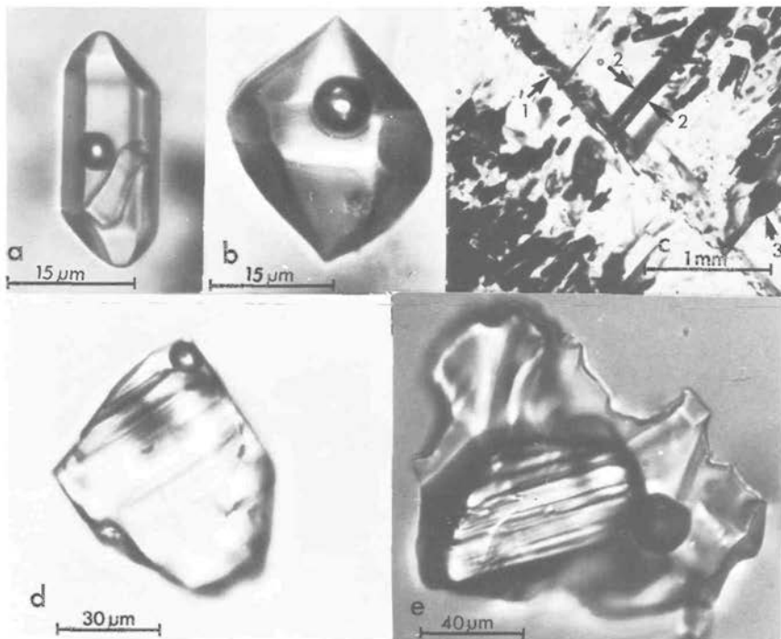
Abb. 10. Fluide Einschlüsse
