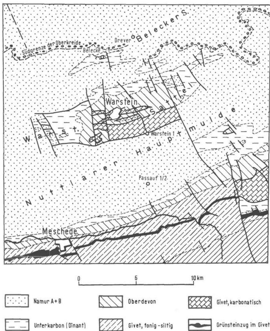
Abb. 1. Übersichtskarte zur Geologie des Warsteiner und Scharfenberger Sattels.
