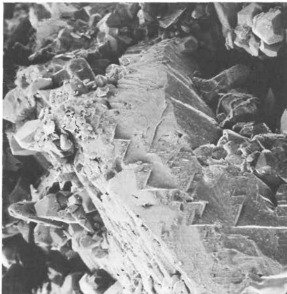
Abb. 12. Teilweise eingewachsene Schwimmkrustenteile auf großem Hohlkristall. Bildbreite 1 mm. (REM-Aufnahme).
